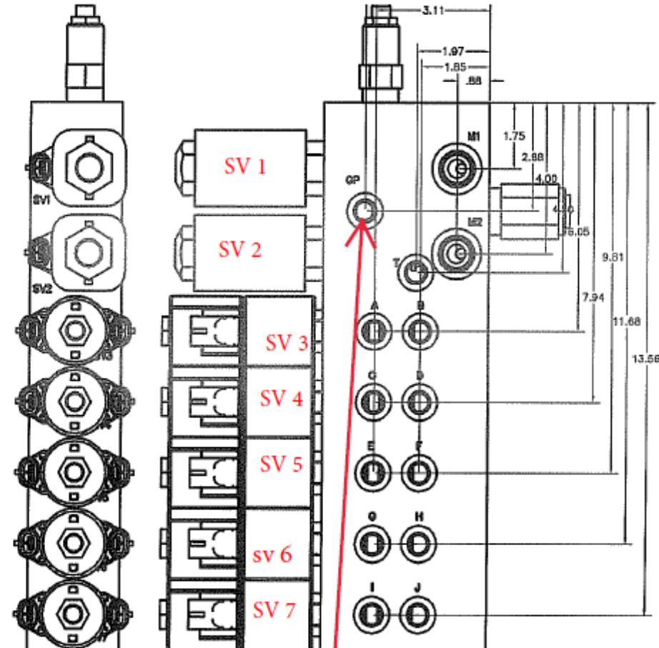
HYDRAULIC TEST POR LOCATION (GP)
