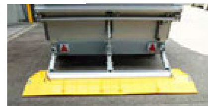
Cinematica finisher ➤ Funzione di ribaltamento migliorata ➤ Scarico semplificato ➤ Ottimizzata per la marcia su strada
